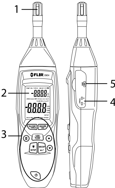
Figure 3.1 Descriptions avant et latérale
