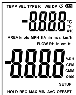
Figure 3.2 Description de l'affichage
